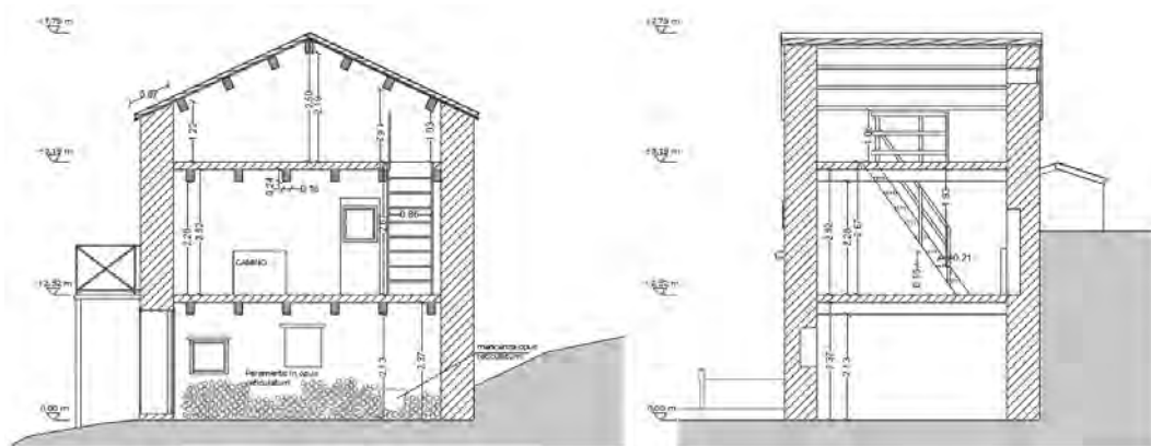
Figura 9: Sezioni caratteristiche della casa colonica.
