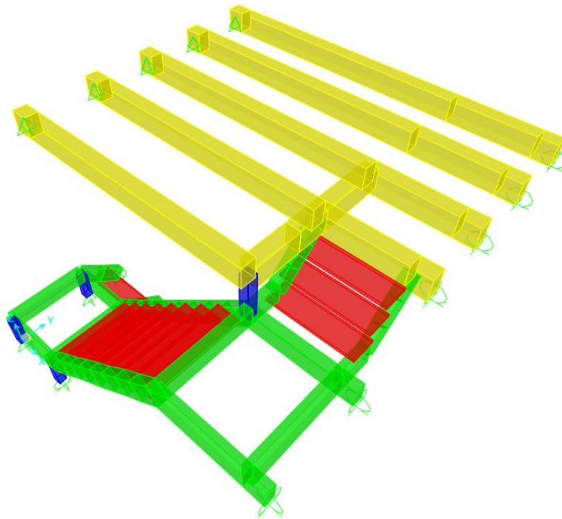
Figura 7. Modello geometrico della scala e del solaio del sottotetto (vista estrusa).
