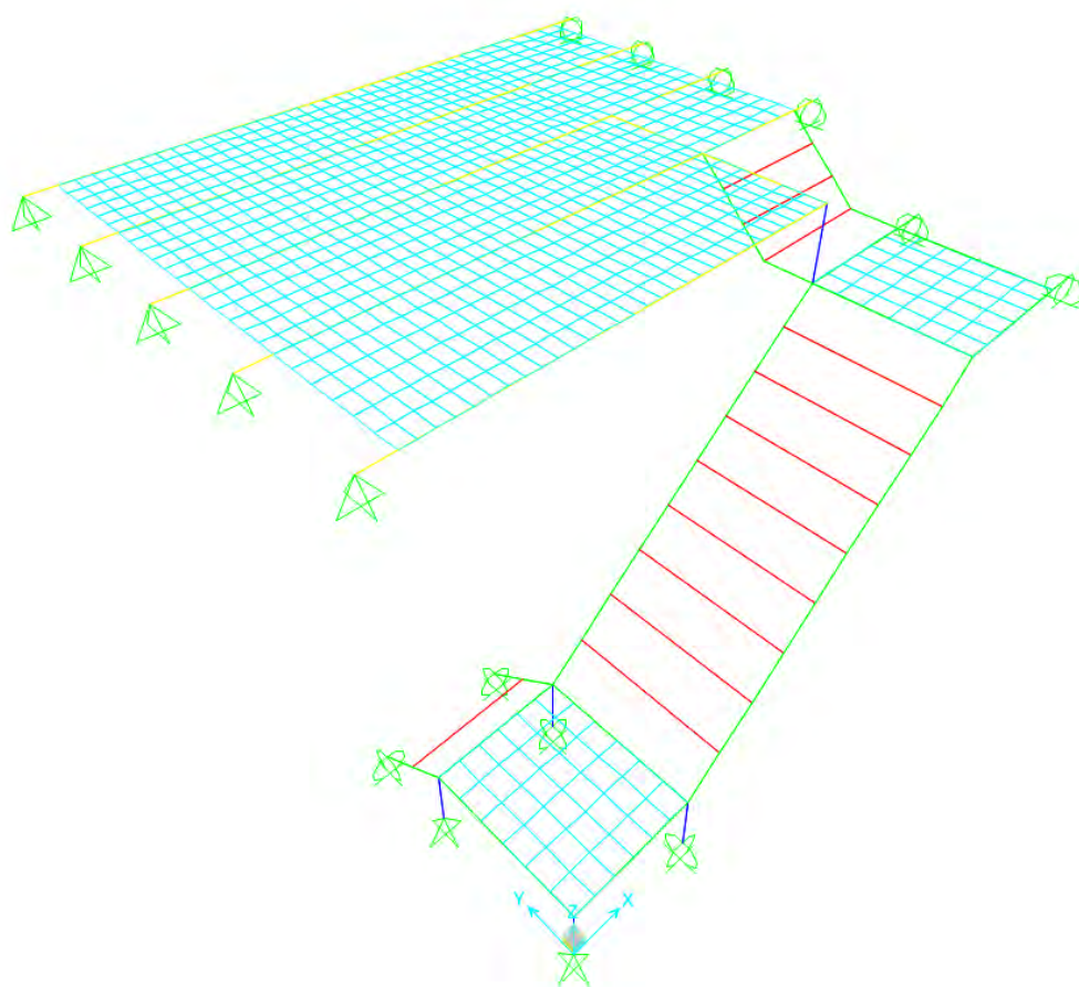
Figura 8. Modello geometrico della scala e del solaio del sottotetto
